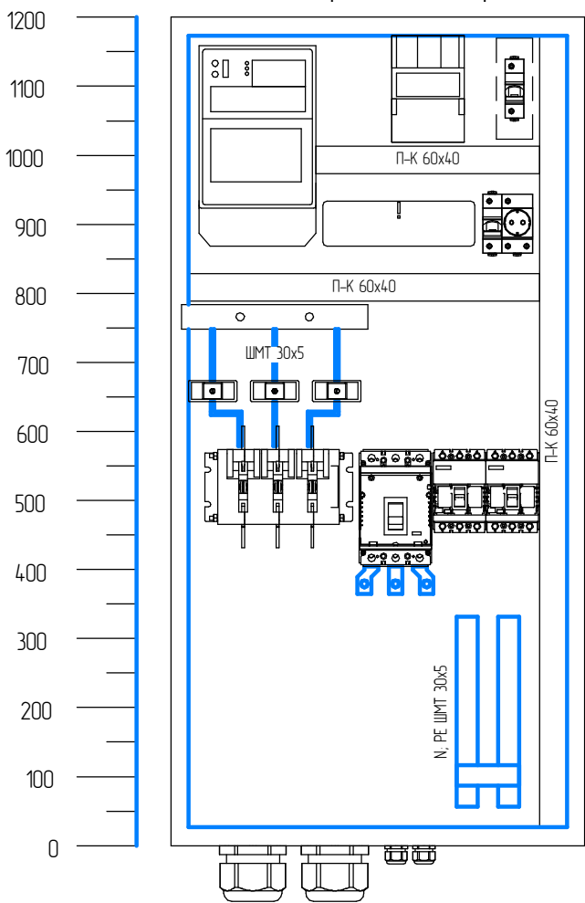
Вид спереди (без двери)
