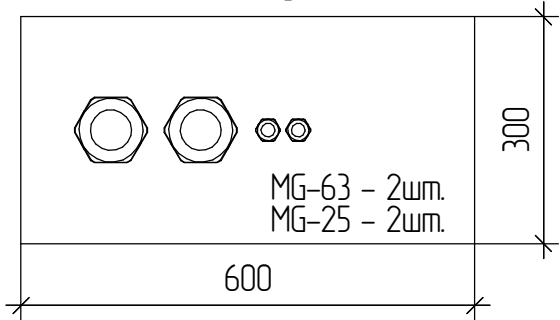
Вид снизу
