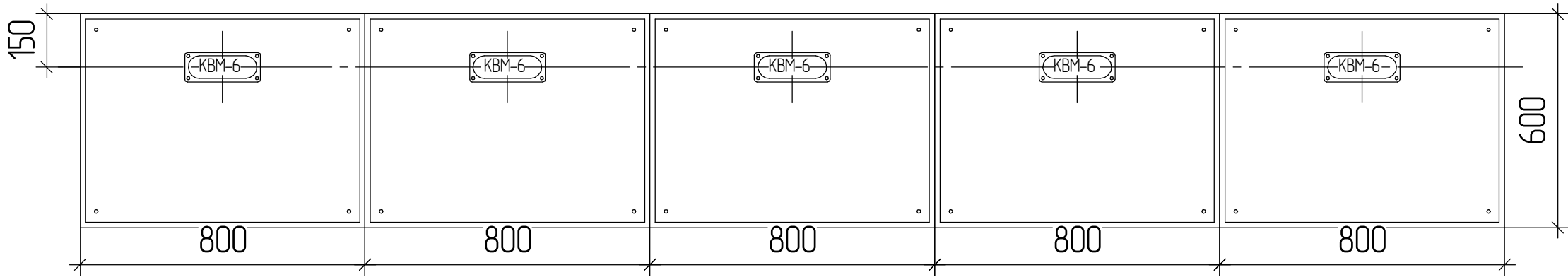
Вид спереди (без дверей)
