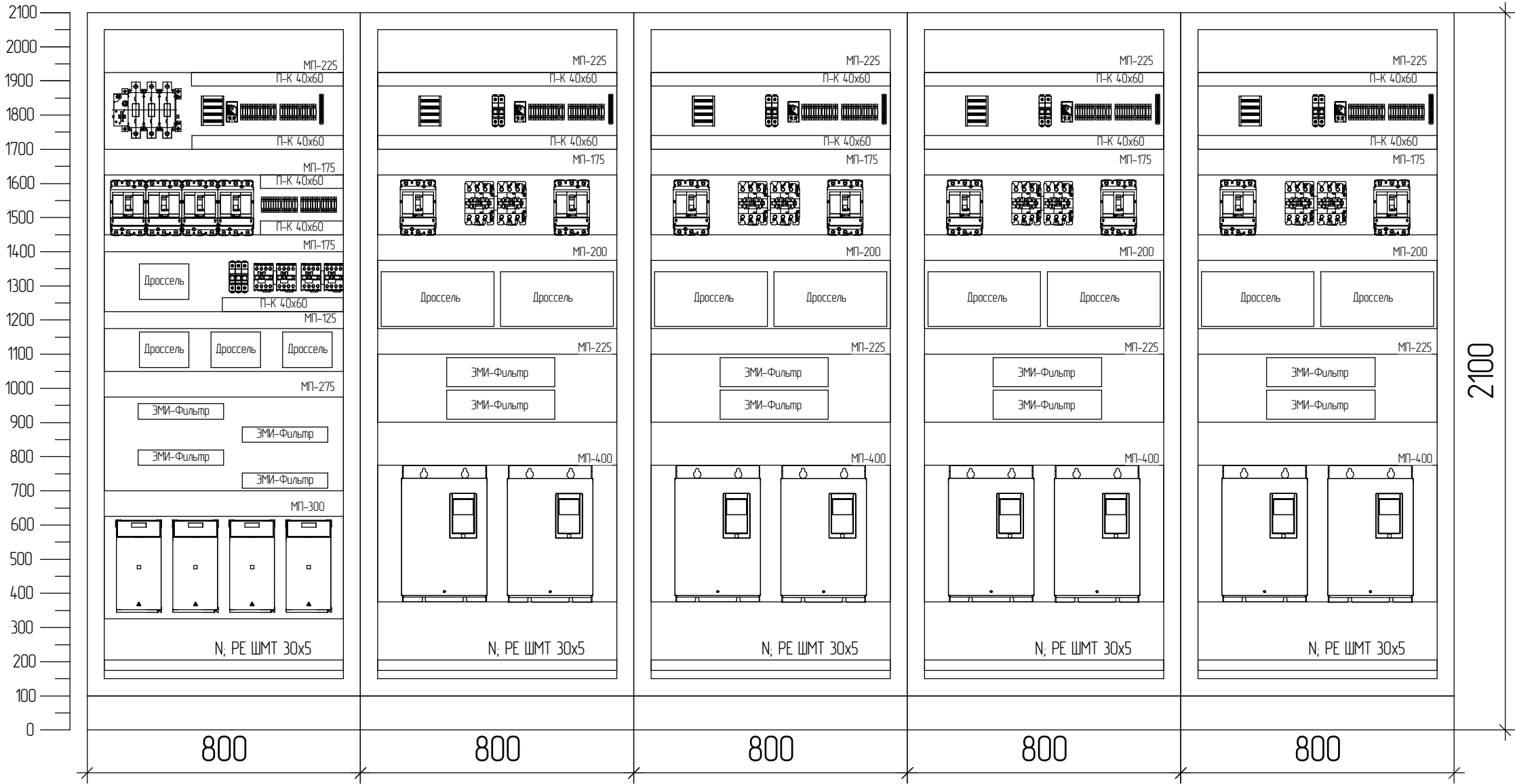
Вид спереди (без дверей)
