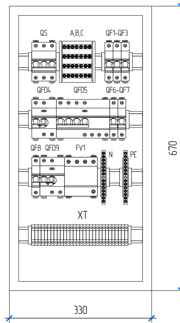
ВИД СПЕРЕДИ (Компоновка)
