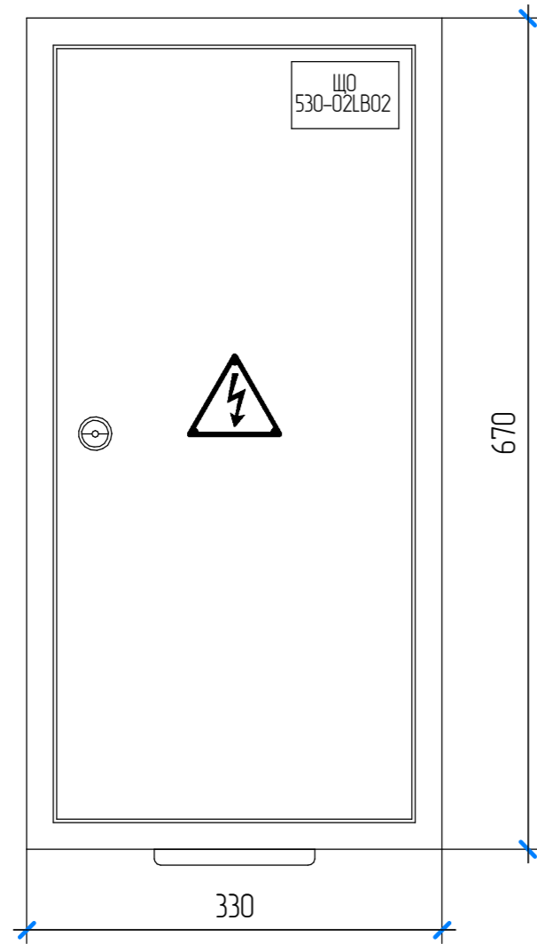
ВИД СПЕРЕДИ
